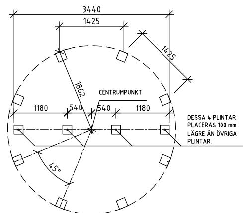
Plintritning
