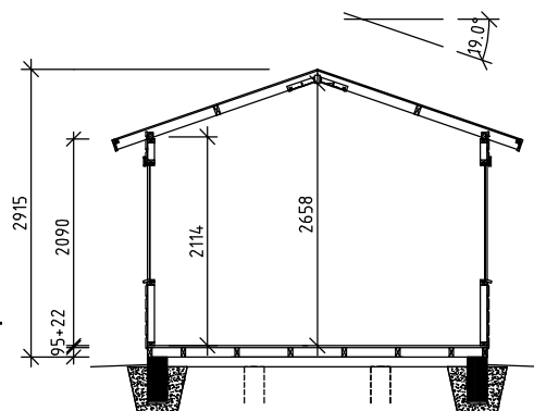
Sektion
