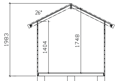
Sektion
