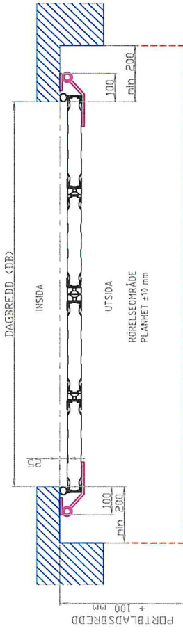
A - A HORIZONTALSEKTION
