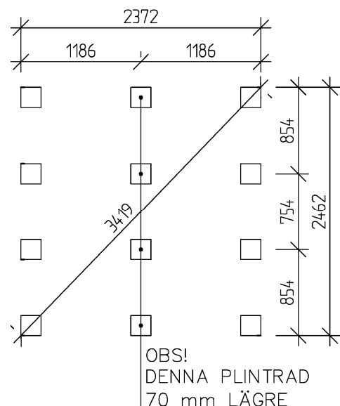
Plintritning
