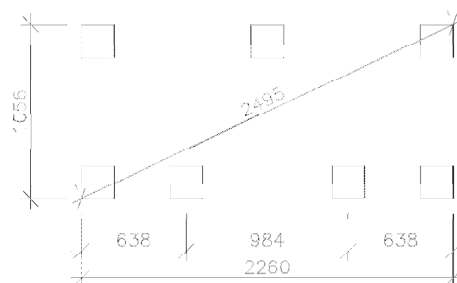
Plintritning
