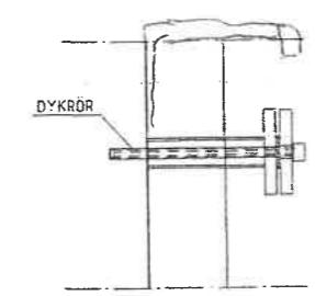
DETALJ TEMP. GIVARE 1:5
