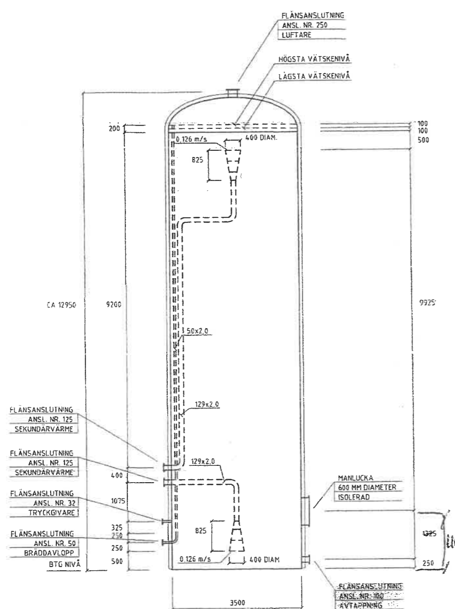
SIDVY A-A VS02-ACK2
