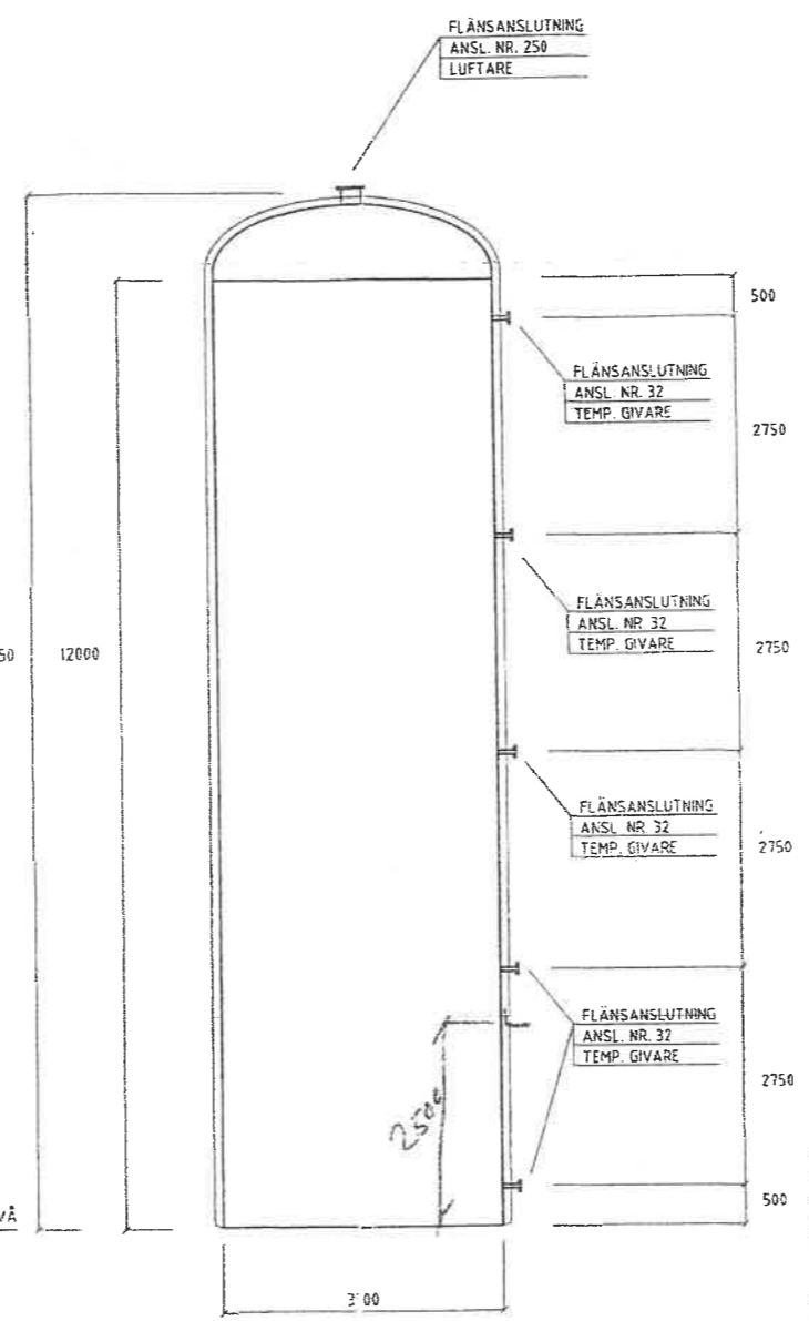
SIDVY B-3 VS02-ACK2
